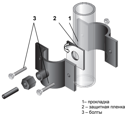
Рисунок 5. Дренажный хомут
